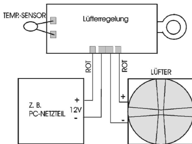
Anschlußbelegung
