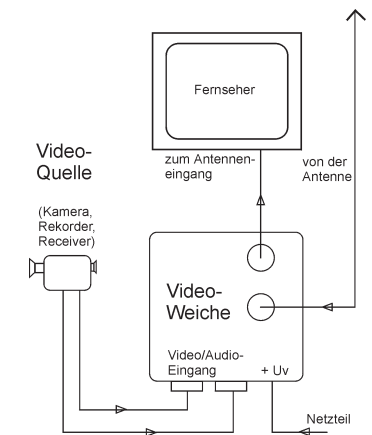
Anschlußskizze
