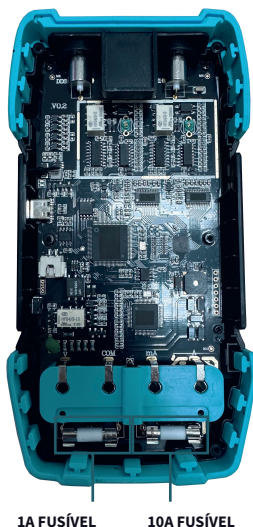
1A FUSÍVEL
