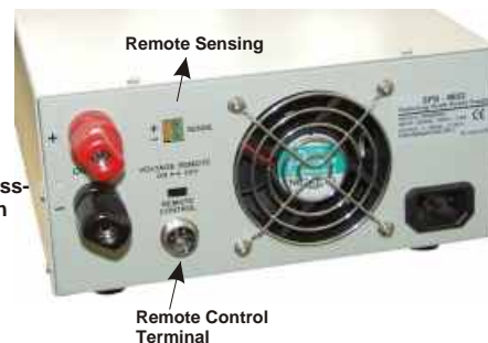
Rückseite SPS9600/9602
